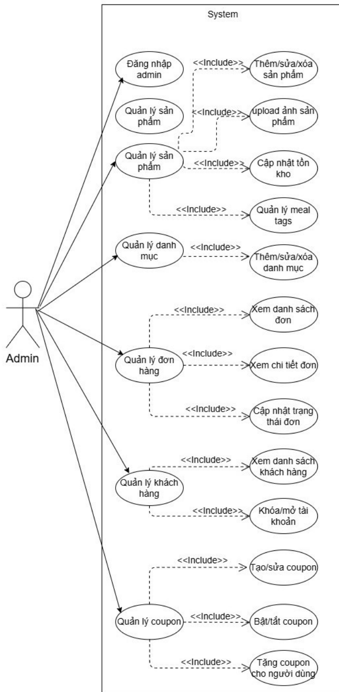
Hình 2.10 Sơ đồ Use Case phân rã của quản trị viên
