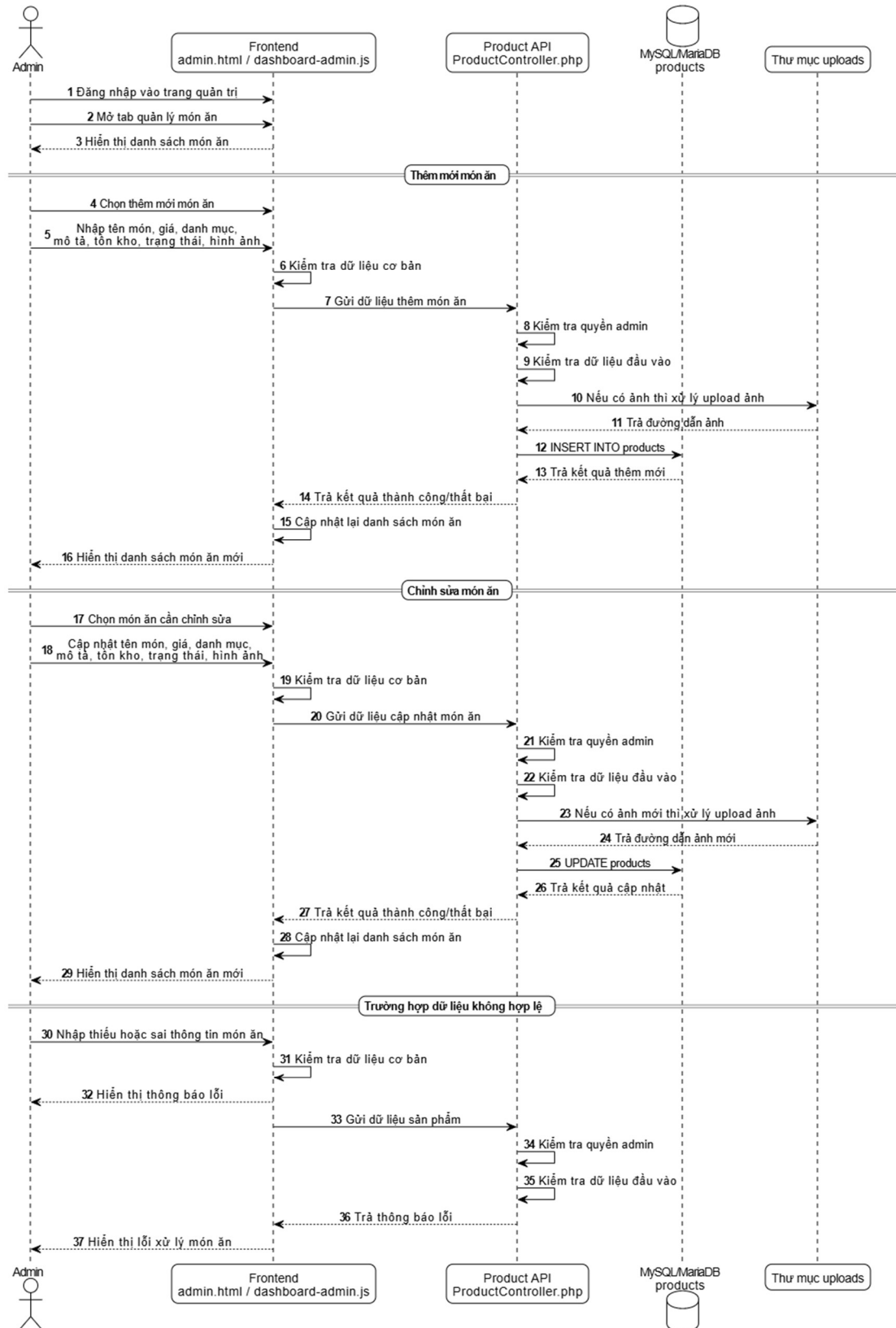
Hình 2.15 Sequence diagram quản lý sản phẩm
