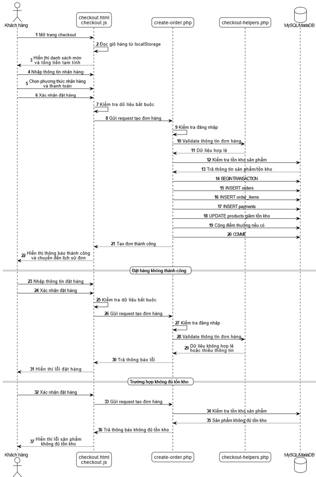
Hình 2.14 Sequence diagram đặt hàng
