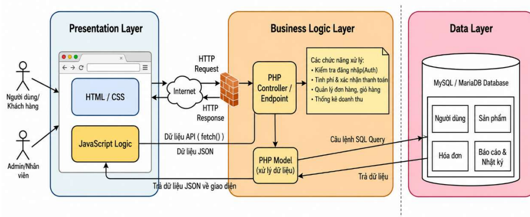
Hình 2.1: Sơ đồ kiến trúc tổng quát của hệ thống đặt
