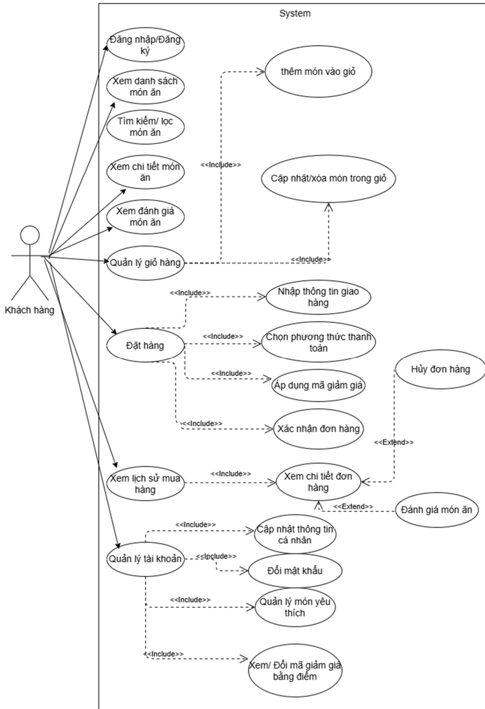
Hình 2.9 Sơ đồ use case phân rã cho khách hàng
