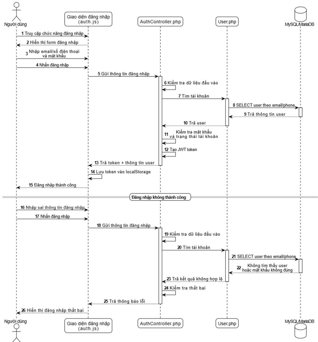
Hình 2.13 Sequence diagram đăng nhập
