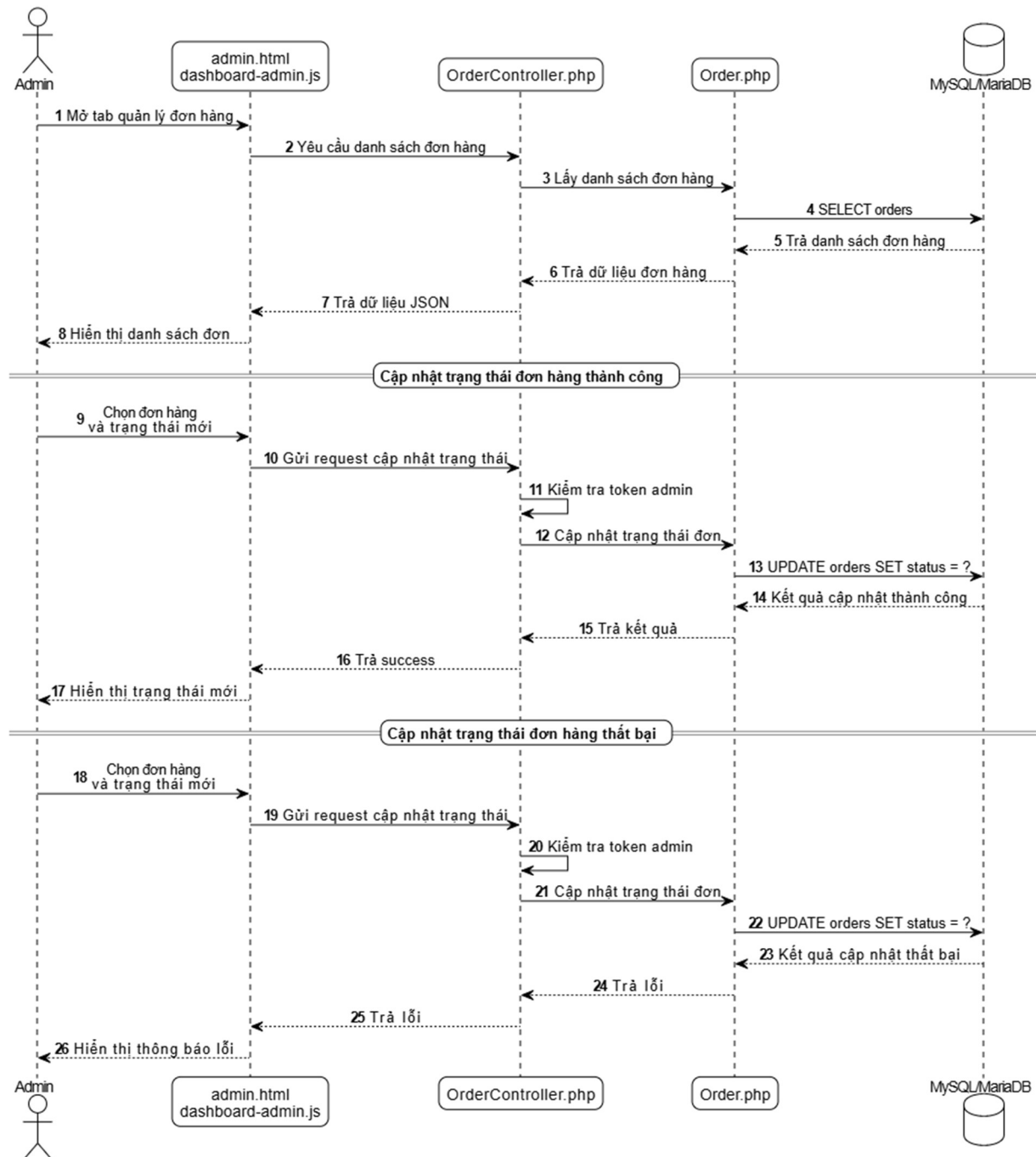
Hình 2.16 Sequence diagram admin cập nhật trạng thái đơn hàng
